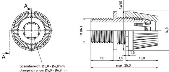
SCHNITT A-A
