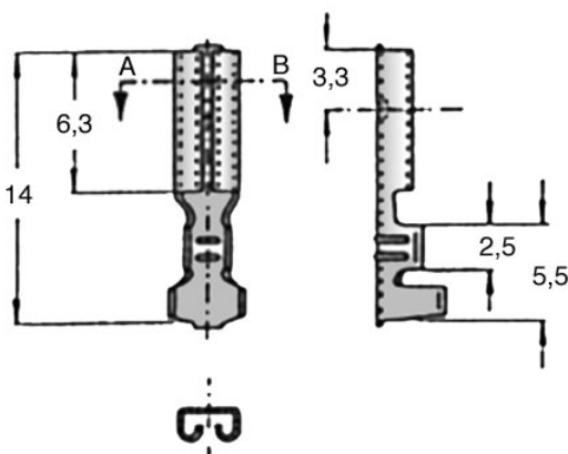
Schnitt A - B
