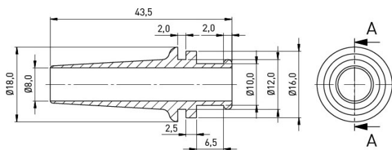
SCHNITT A-A
