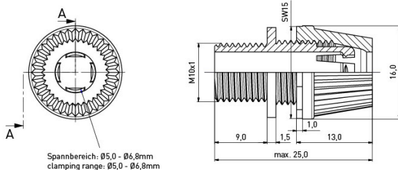
SCHNITT A-A
