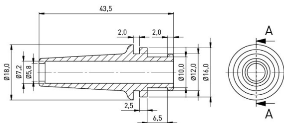
SCHNITT A-A
